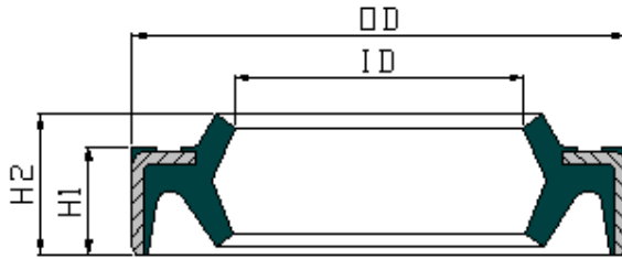
YH77 TYPE
