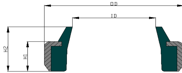
YH88 TYPE
