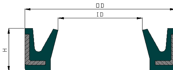
YH63 TYPE
