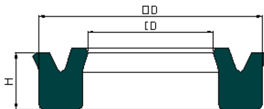
YH55 TYPE
