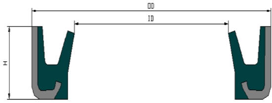
YH66 TYPE
