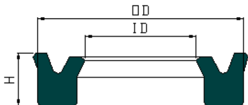
YH21 TYPE
