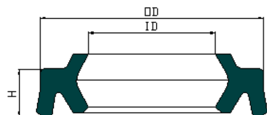
YH51 TYPE
