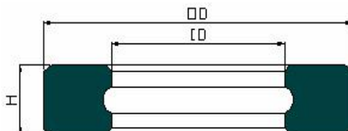
YH57 TYPE
