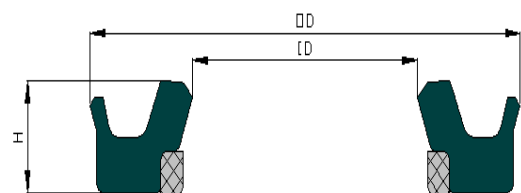
YH25 TYPE
