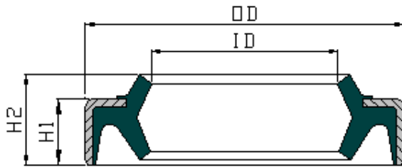
YH78 TYPE
