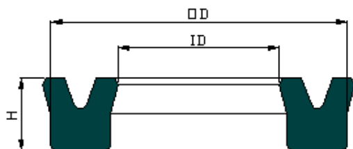
YH33 TYPE
