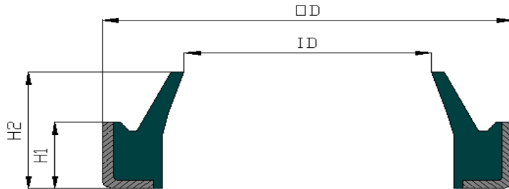
YH78 TYPE
