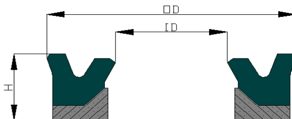
YH59 TYPE
