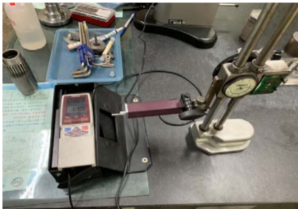
Surface Roughness Tester (Mitutoyo)
